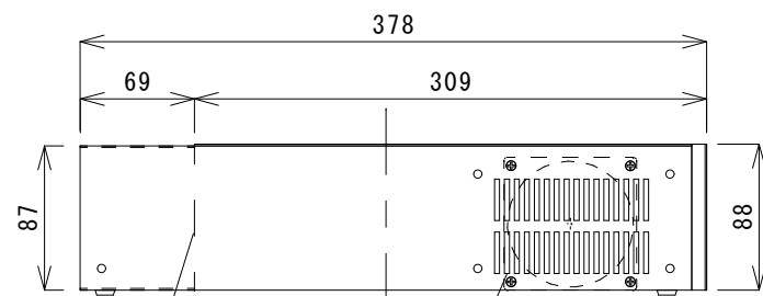
【左側面】 通気孔 内部、ファンあり
