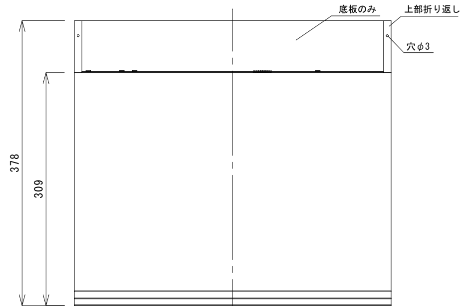
【上面】
