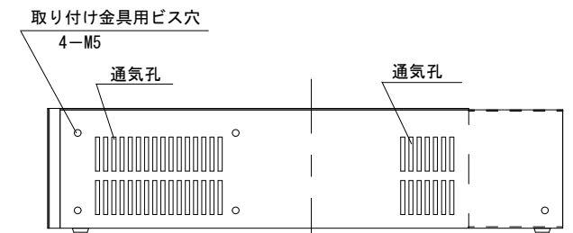
【右側面】
