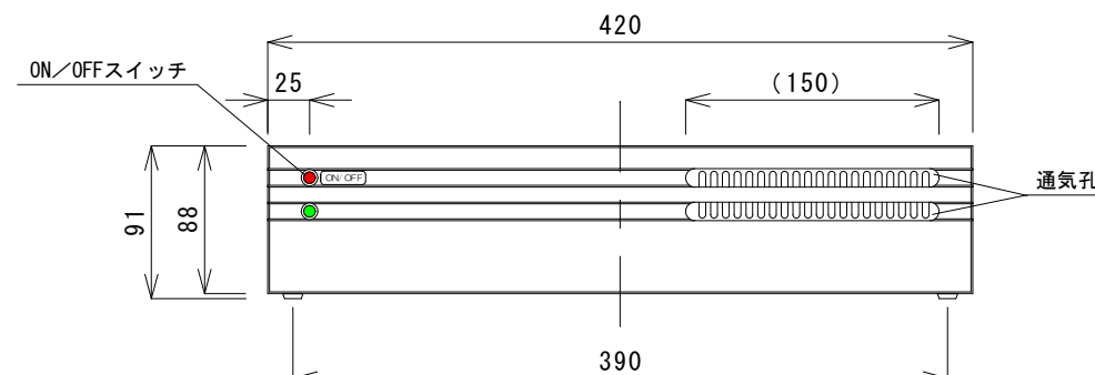
【正面】
