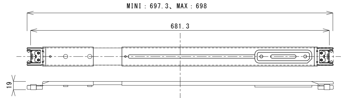
【付属ラックマウントレール】
