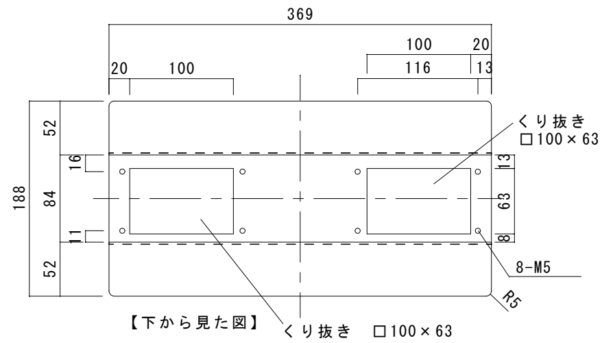
・縦置き用スタビライザー寸法図
