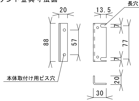
・ラックマウント金具寸法図
